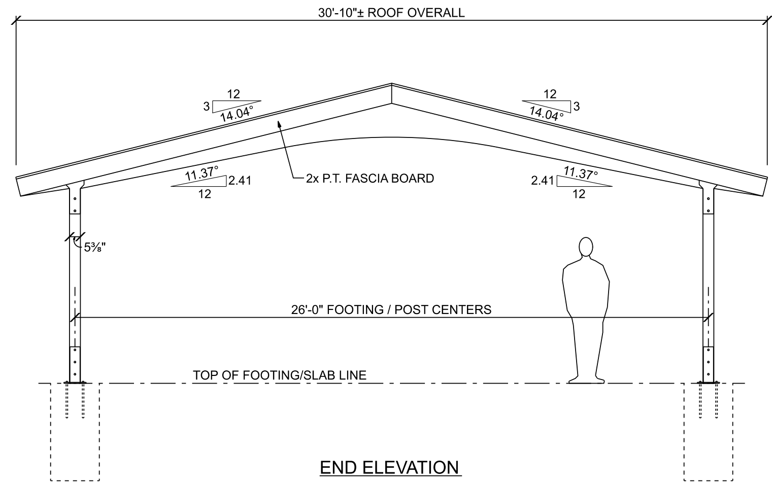
END ELEVATION
