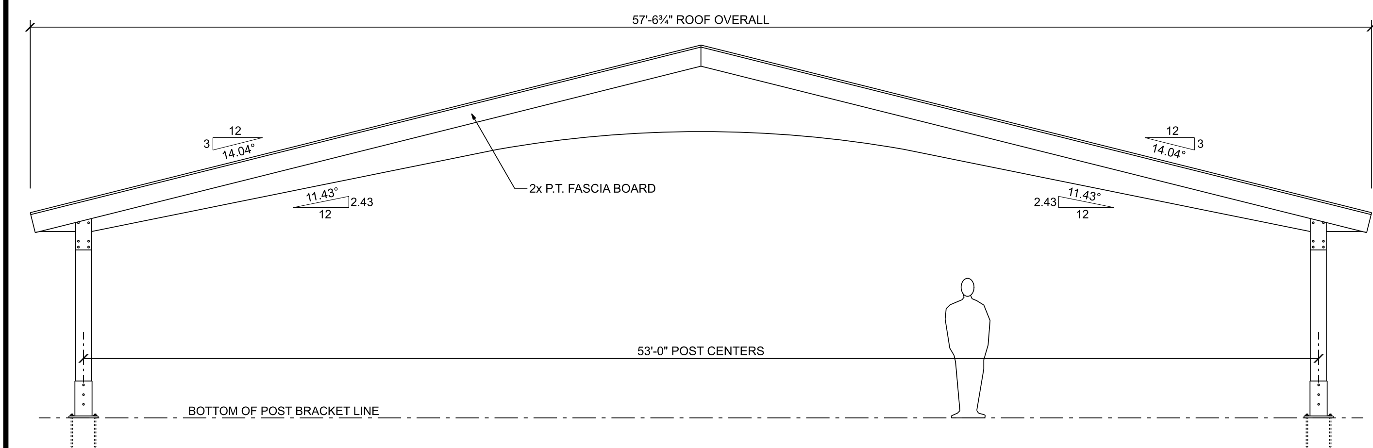
END ELEVATION
